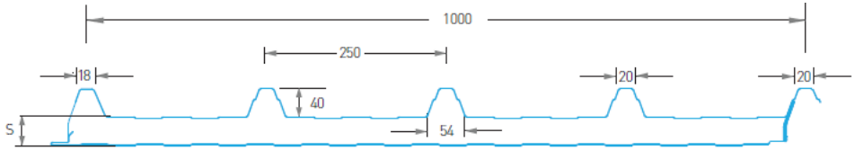
DISEGNO TECNICO DEL PANNELLO SANDWICH
