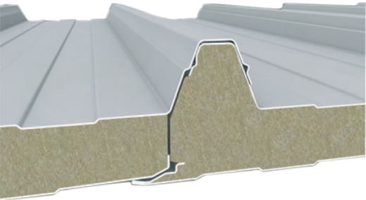
DETTAGLIO DEL PANNELLO FONOASSORBENTE
