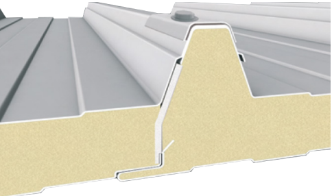
DETTAGLIO DEL PANNELLO SANDWICH
